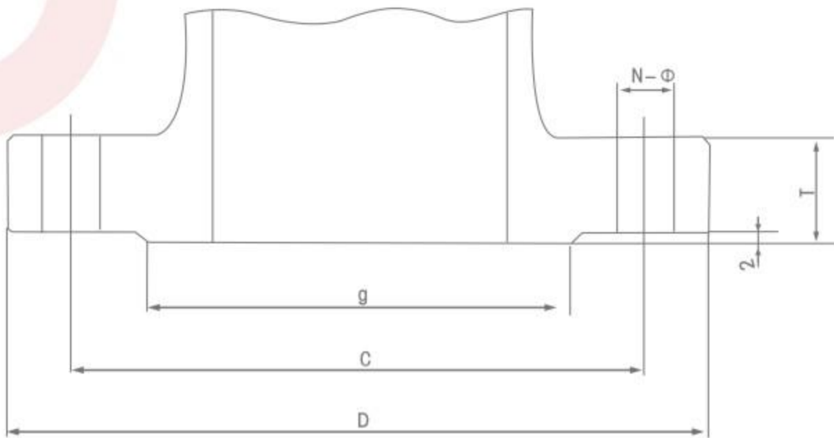
GB/T PN16 / PN40(RF)steel
